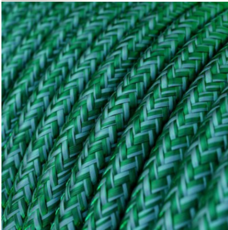
Textilkabel, smaragdgrün glänzend - Das Original von Creative-Cables - RM33 rund 3x0,75mm
